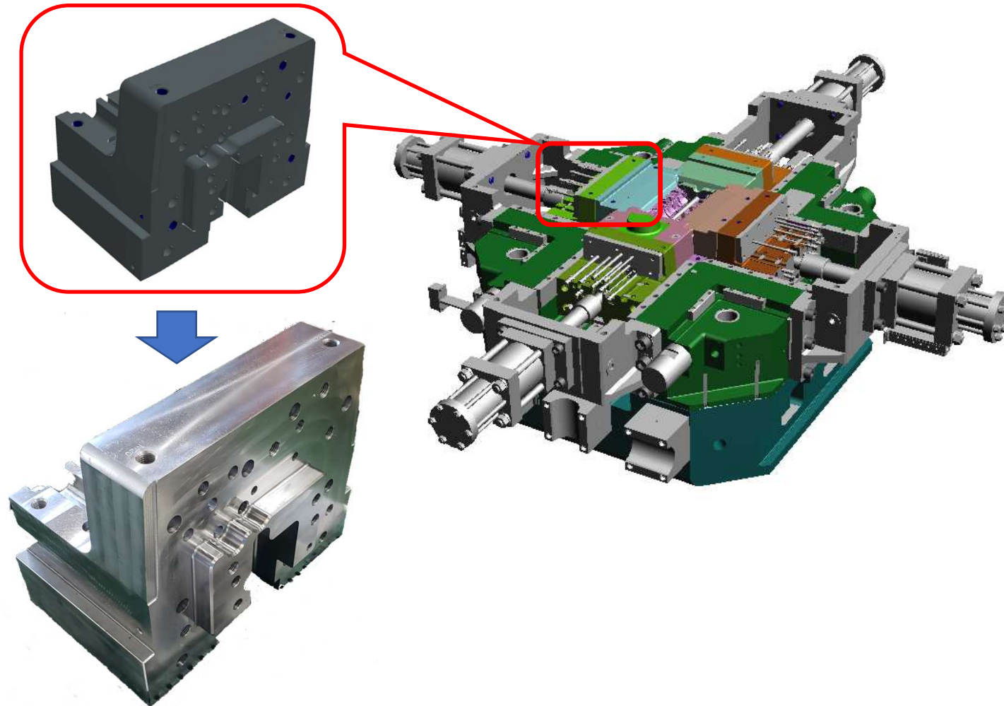
スライドコアホルダー
